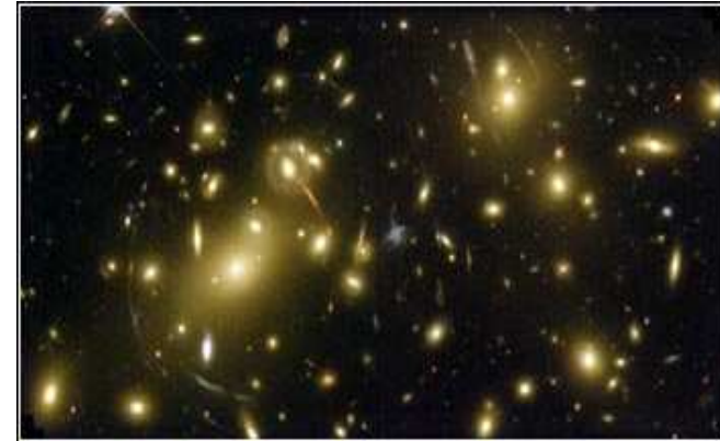
Cada ponto luminoso é uma galáxia
