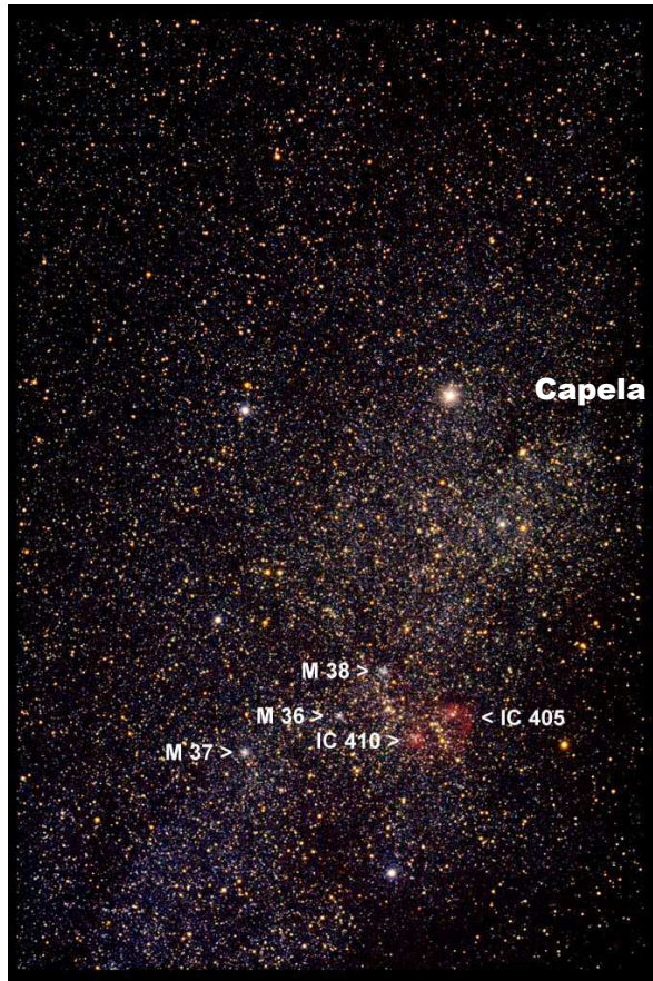
Constelação do Cocheiro Capela é a mais brilhante
