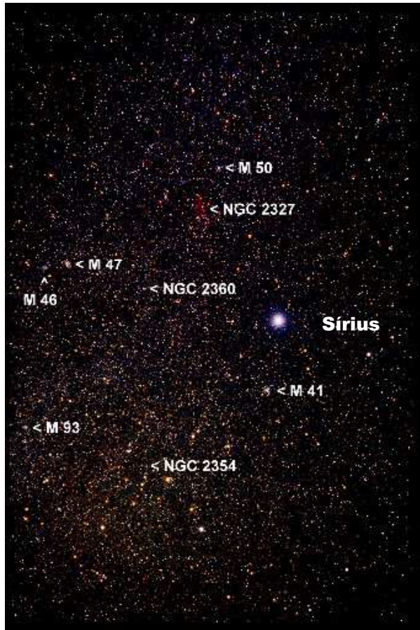
Constelação do Grande Cão Sirius é a mais brilhante
