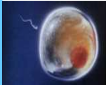
Fecundação
