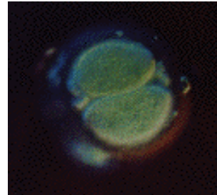
30 horas
